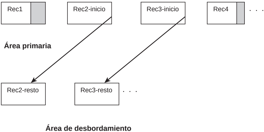
FIGURA A.4(c) Uso de registros con longitud fija primaria y de desbordamiento
