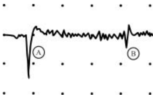
Fig. 10.9. Esquema de la actividad espontánea en la EMG. Onda aguda positiva (A) por convención la deflexión positiva es hacia abajo, y una fibrilación trifásica pequeña (B). Estos hallazgos sugieren deservación activa con despolarización espontánea de las fibras musculares aisladas deservadas.
