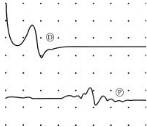
Fig. 10.7. Esquema de la neuroconducción del bloqueo de la conducción con dispersión temporal. La velocidad de barrido es de 5 milisegundos/división y la sensibilidad es de 1 mV/división. Cuando el potencial de acción compuesto motor de la estimulación distal (D) es comparado con el de la estimulación proximal (P), se constata una caída de más de 50 % de la amplitud. La duración de la onda se incrementa, al igual que la complejidad. Estos hallazgos sugieren desmielinización de los nervios entre los sitios de estimulación, con bloqueo de la conducción en la mayoría de los axones motores. También existe incremento de la variabilidad en el rango de los tiempos de conducción axonal causando un incremento de la duración de la onda (dispersión temporal).
