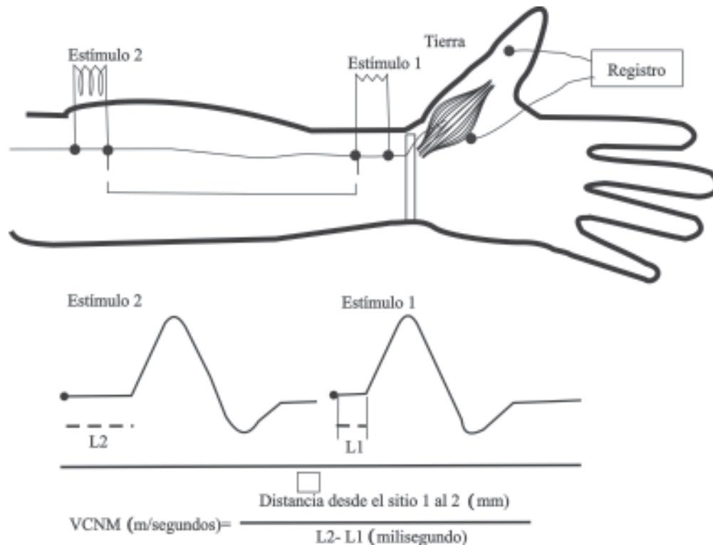
Fig. 10.4. Técnica general para estudiar la conducción nerviosa motora. Se ejemplifica con el nervio mediano estimulado a nivel de la muñeca o en la flexura del codo; el potencial de acción muscular derivado puede registrarse como la diferencia de potencial entre un electrodo de superficie, sobre la eminencia tenar y un electrodo de referencia más distal. El trazado primero representa el artefacto producido por el estímulo. La amplitud se mide desde la línea de base hasta el pico negativo. Las latencias A y B son denominadas latencias distal y proximal, respectivamente, y son medidas desde el estímulo hasta el inicio de la respuesta. El método para calcular la VCNM se representa abajo.
